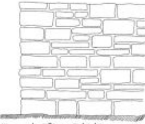
Unregelmäßiges Schichtenmauerwerk
